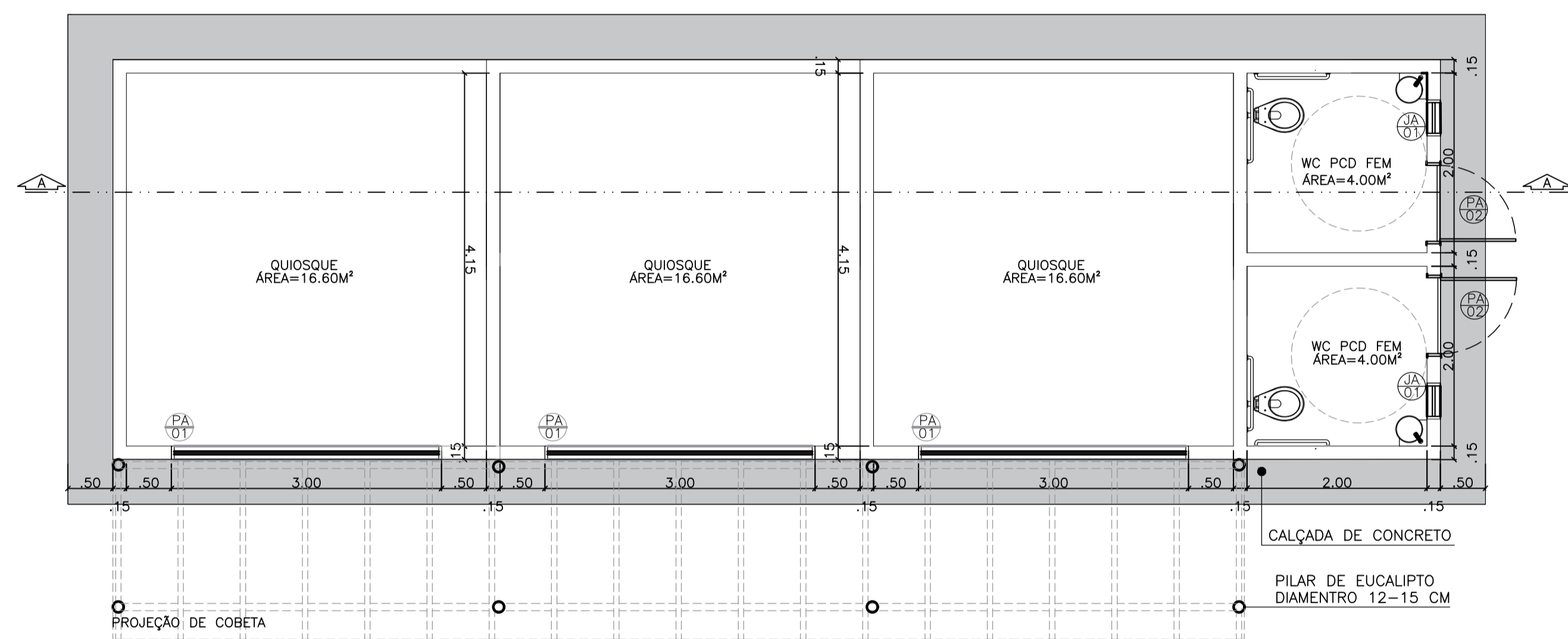
PLANTA BAIXA TÉCNICA QUIOSQUE esc 1:50
