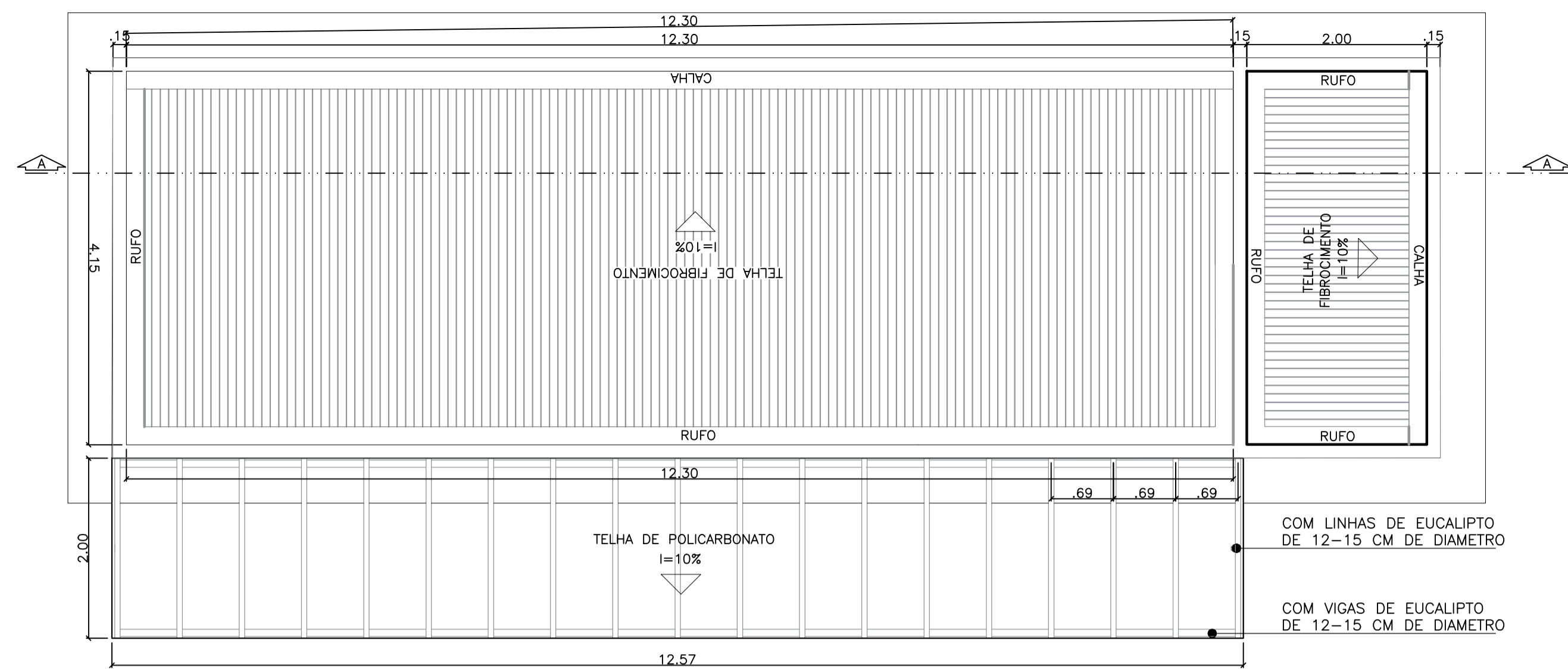
PLANTA DE COBERTA QUIOSQUE esc 1:50
