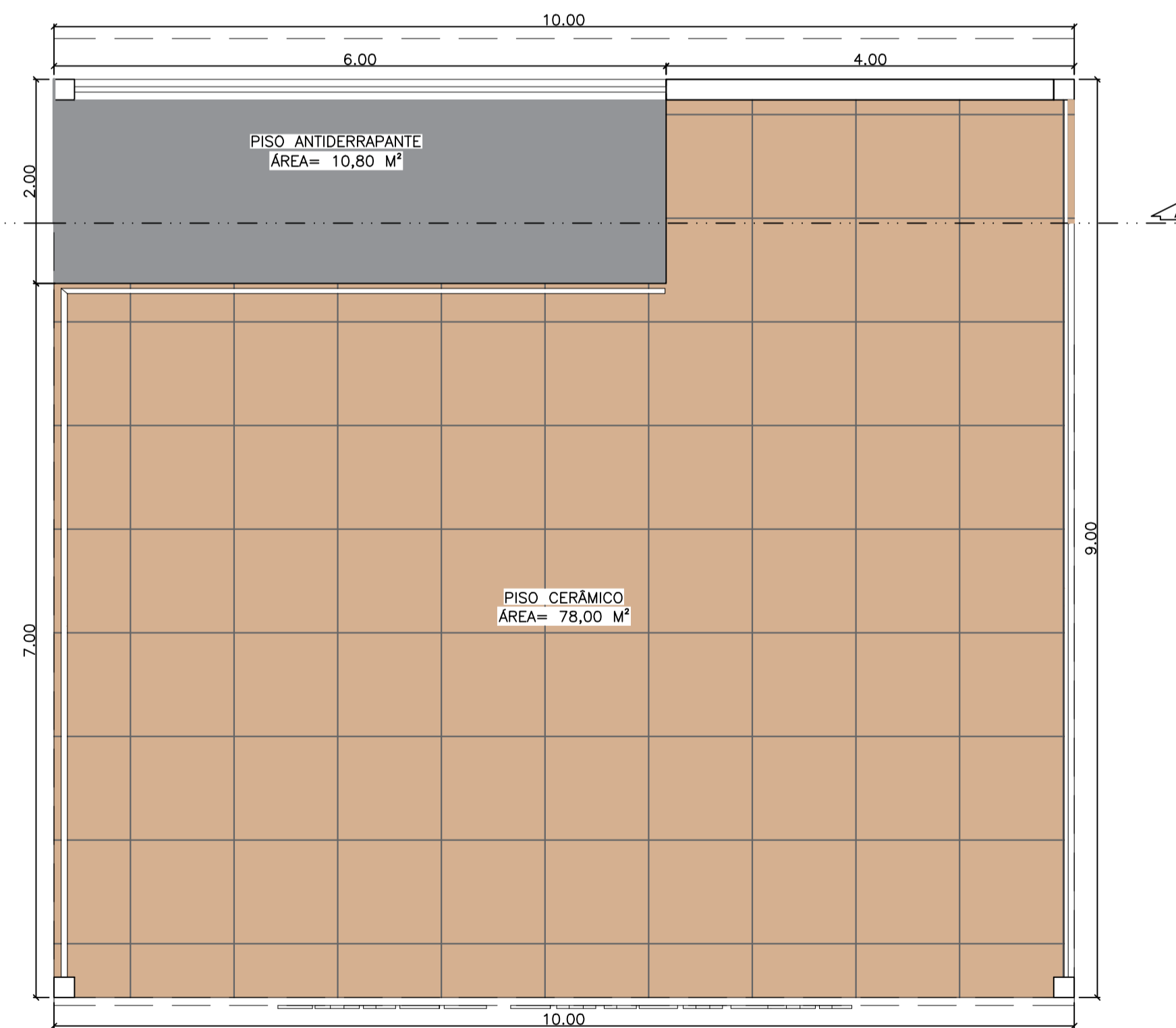
PLANTA DE PISO - PALCO CULTURAL esc 1:50
