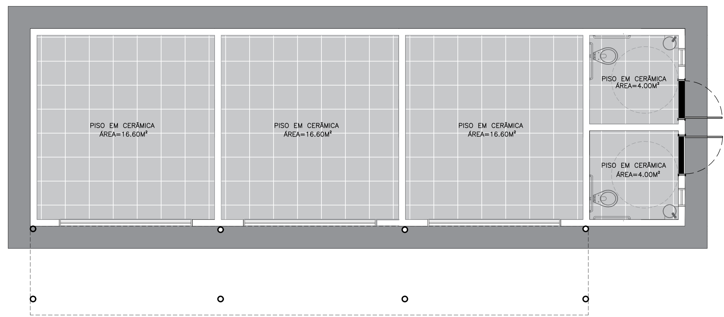
PLANTA DE PISO esc 1:50
