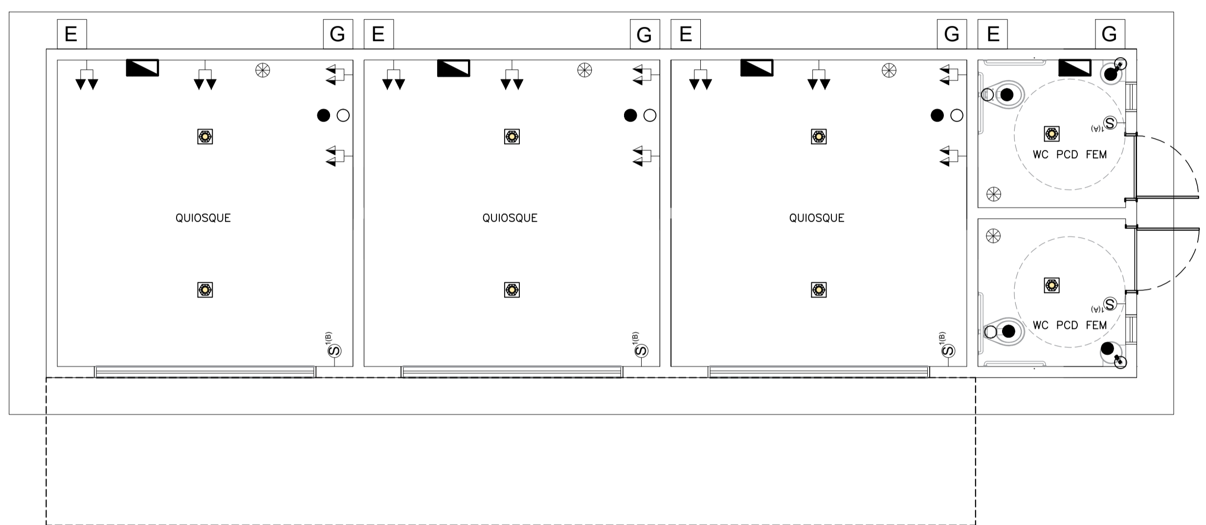
PLANTA DE PONTOS ELÉTRICOS E HIDRÁULICOS esc 1:50
