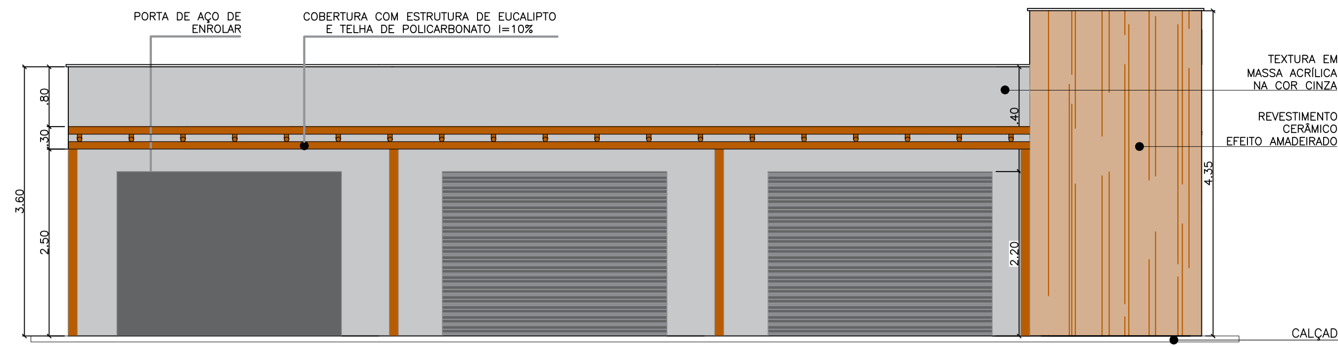
FACHADA QUIOSQUE esc 1:50
