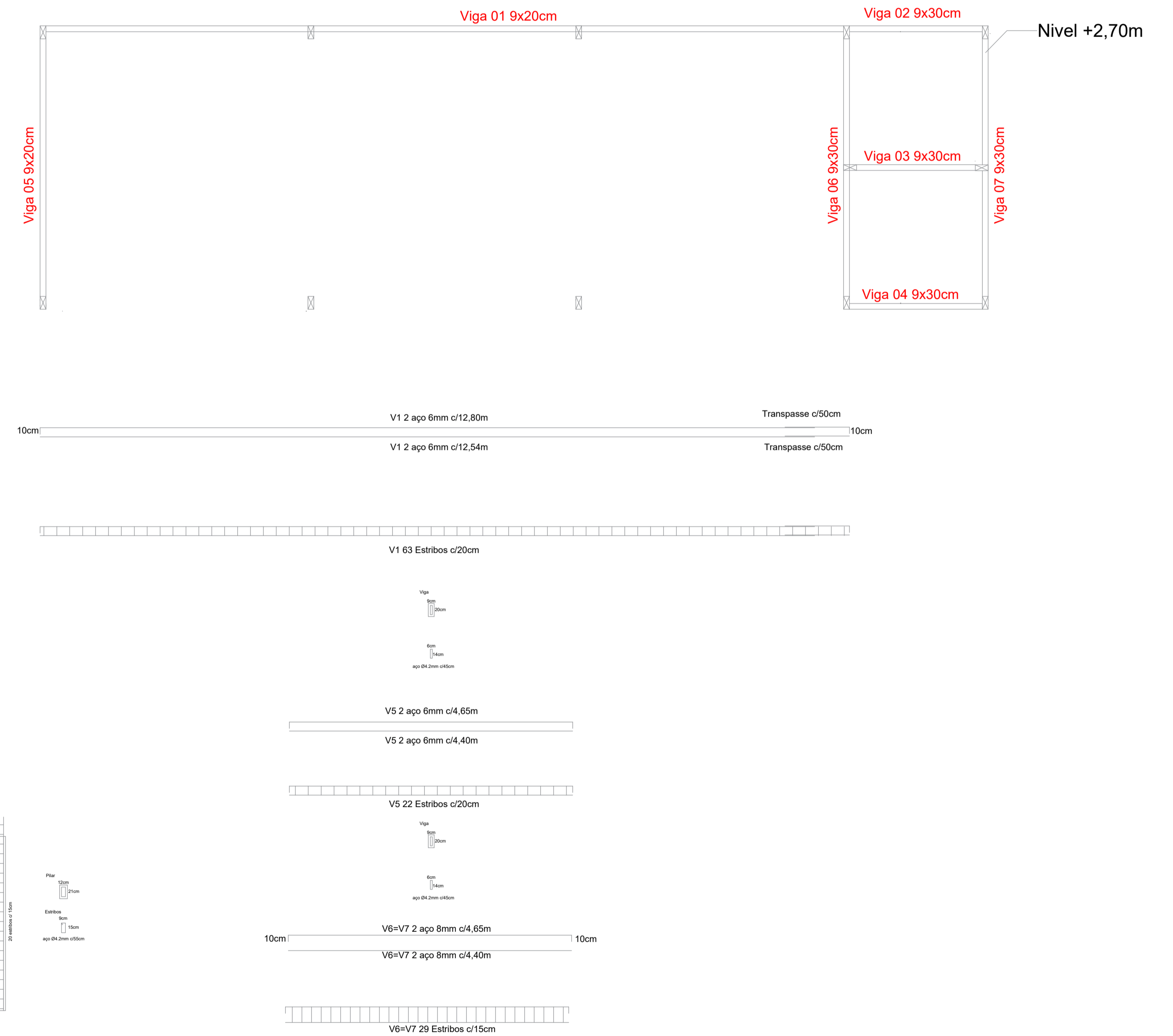
Planta de viga térreo
