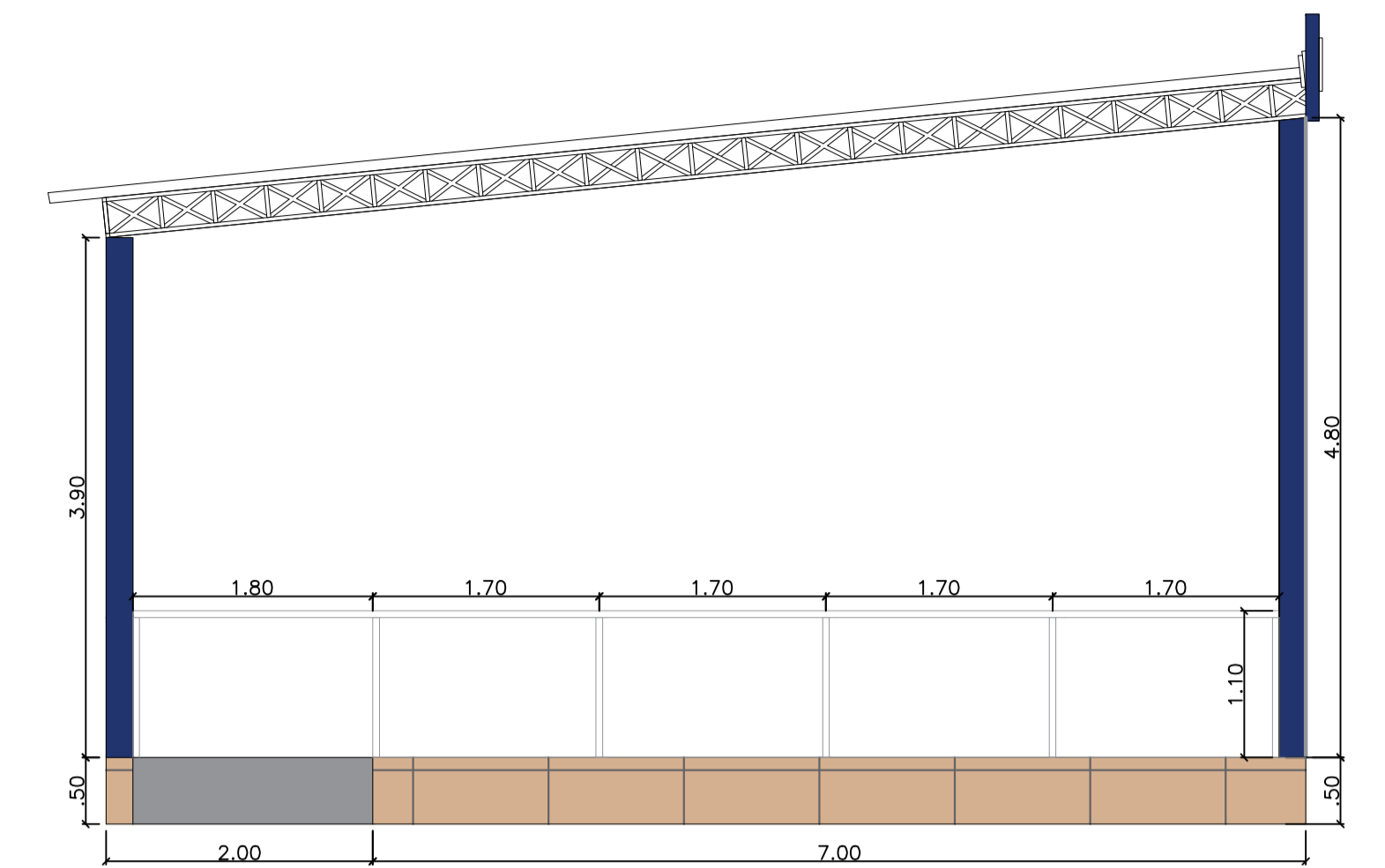
VISTA LATERAL 2 - PALCO CULTURAL esc 1:50
