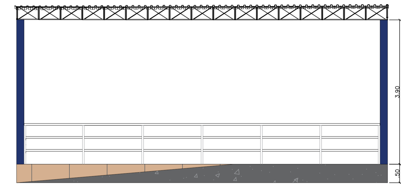
CORTE AA - PALCO CULTURAL esc 1:50
