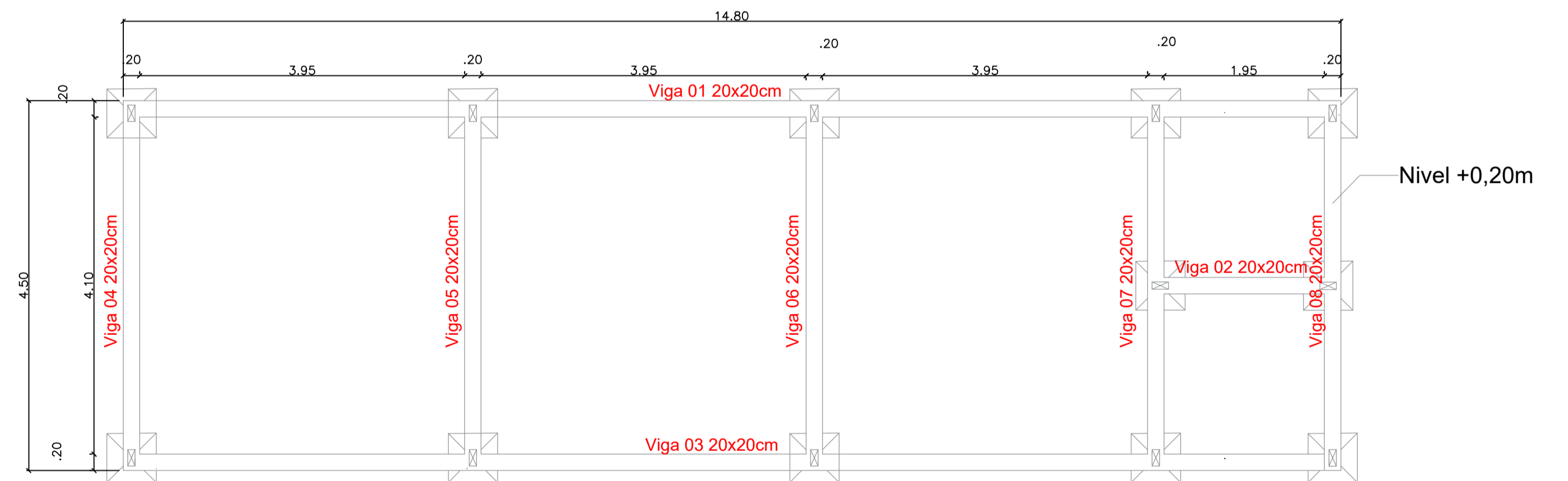
Planta de vigas baldrame dos quiosque
