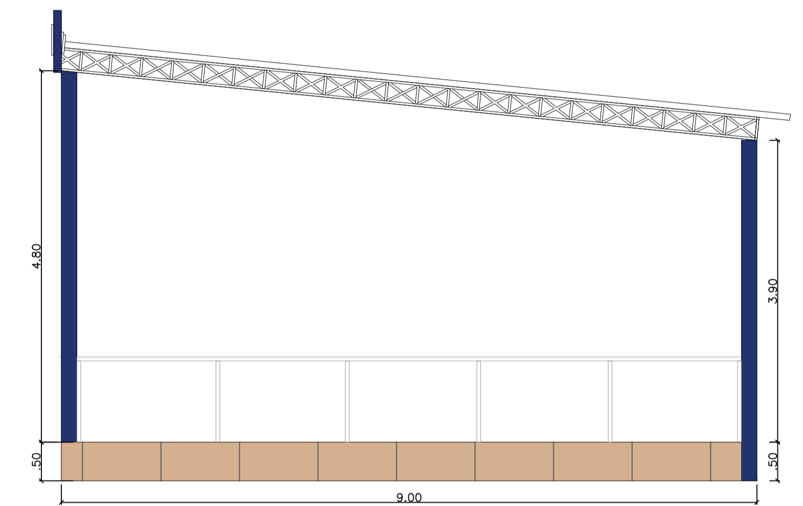
VISTA LATERAL 1 - PALCO CULTURAL esc 1:50
