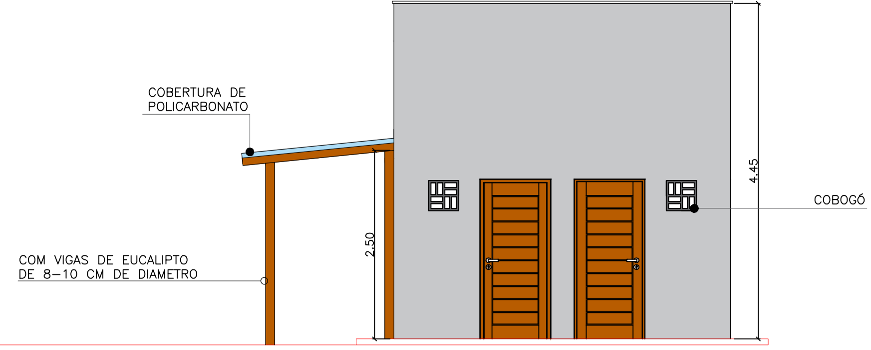
FACHADA LATERAL QUIOSQUE esc 1:50
